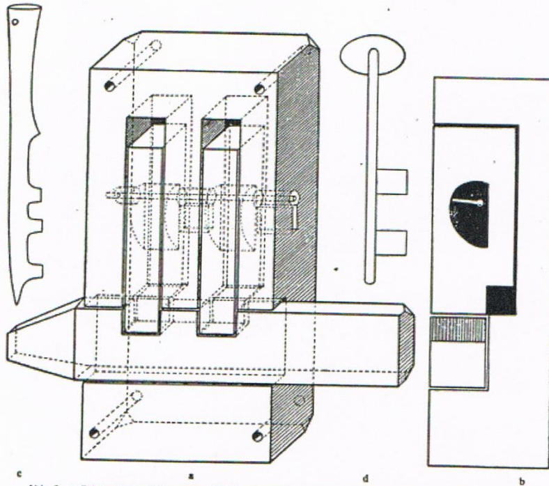
Abb. 3. a Schematische Skizze eines Fallriegelschlosses, dessen Klötzchen mit Drehschlüssel zu heben. b Querschnitt durch das Schloß. c Drehschlüssel aus Holz. d Drehschlüssel aus Eisen.
